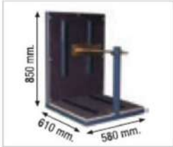
PLATAFORMA PLACAS SOLARES SOLAR PANELS PLATFORM
